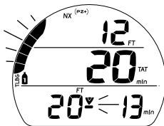
Fig. 67 - VIOLAZIONE DIFFERITA 1 PRINCIPALE (durante l'attivazione dell'allarme acustico)
