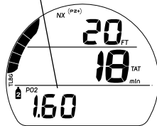
Fig. 74 - ALLARME PO2 (in Decompressione)
