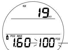
Fig. 17 - IMPOSTAZIONE FO2 GAS 2
