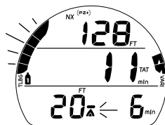
Fig. 61 - INGRESSO DE-COMPRESSIONE (durante l'attivazione dell'allarme acustico)
