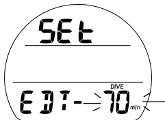
Fig. 22 - IMPOSTAZIONE ALLARME EDT
