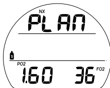
Fig. 8B - SCHERMATA INTRODUTTIVA PLAN (Gas 1 impostato su Nitrox)
