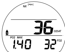
Fig. 6 - NORM SURF ALT 3 (solo se si impiega Nitrox)
